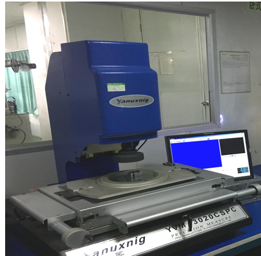
Двухкоординатный измеритель
